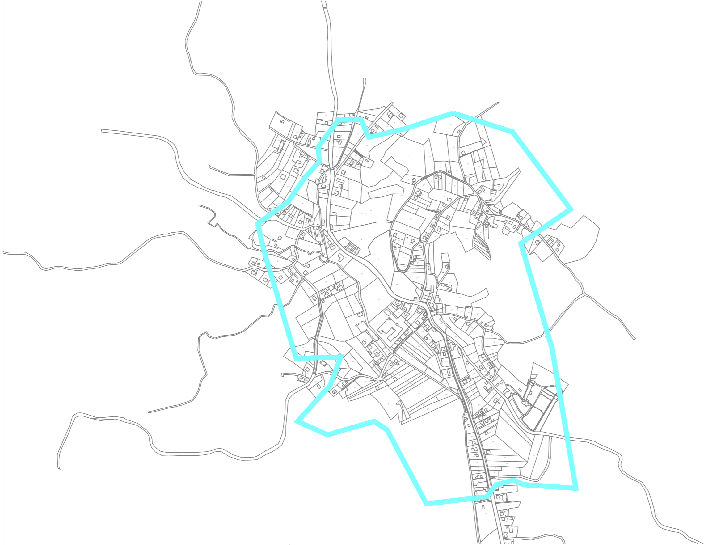
Zona obuhvata FTTH_DONJA PUŠĆA - proširenje obuhvata Donja Pušća 2
