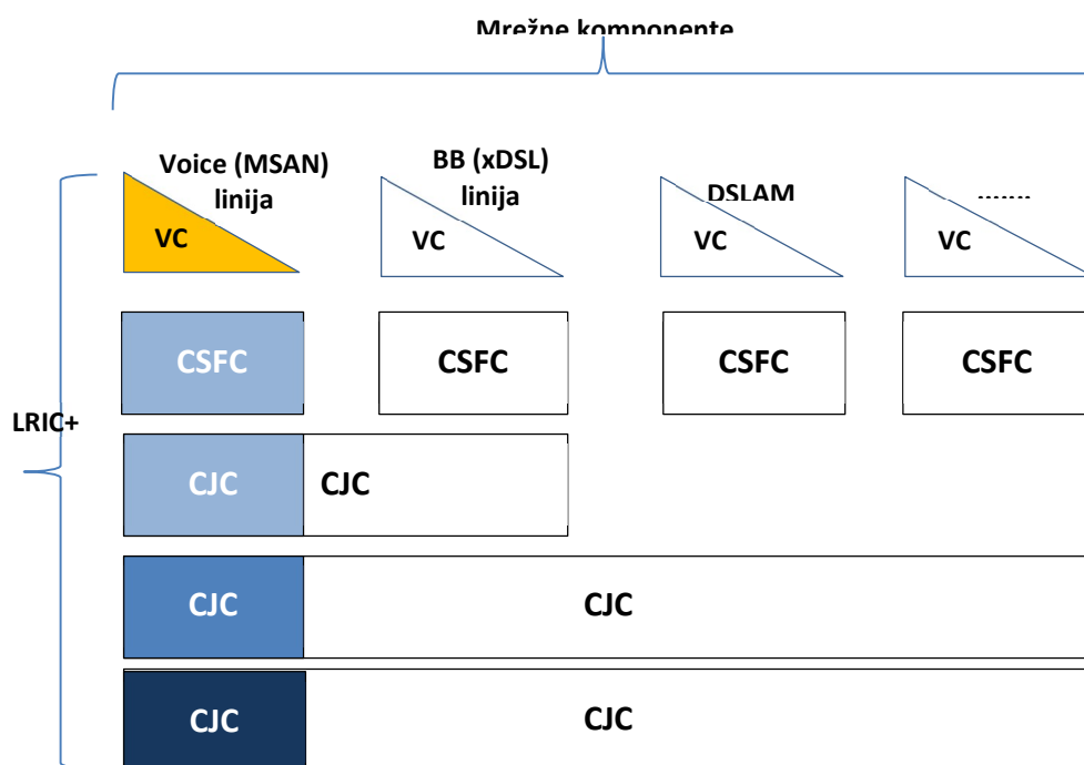
Slika 1.5 LRIC+
