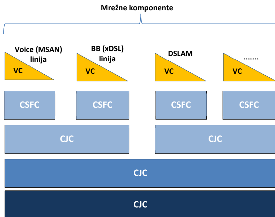
Slika 1.3 Troškovni koncepti
