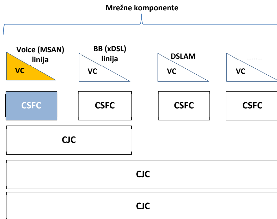
Slika 1.4 LRIC
