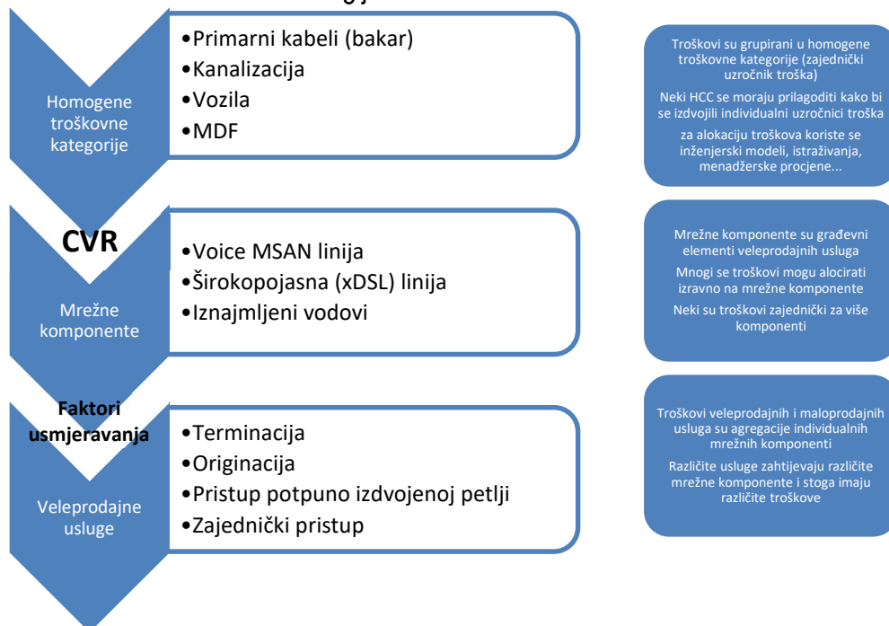
Slika 1.1 LRIC metodologija
